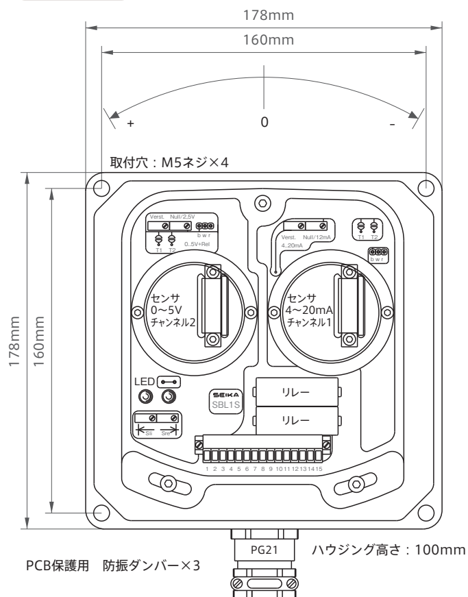
外形寸法図
