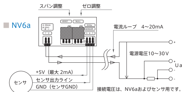
接続図
