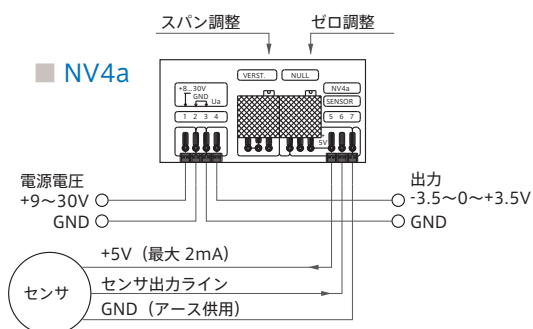
接続図
