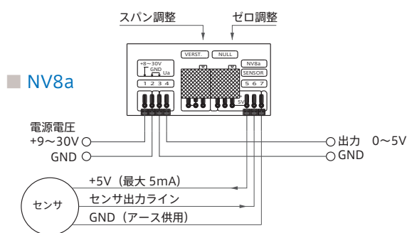
接続図
